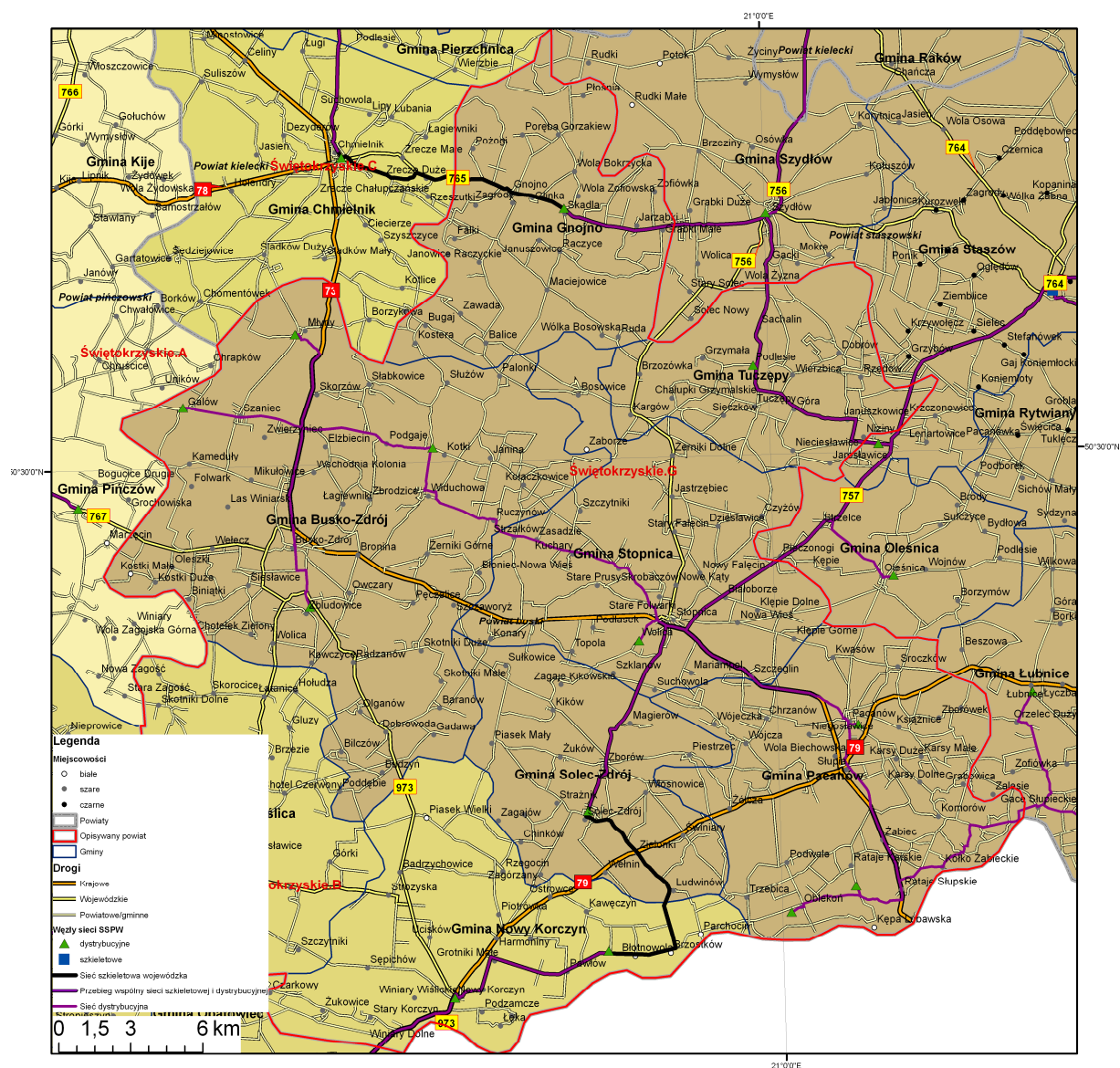
Rysunek 21 Wizualizacja przebiegu sieci szkieletowej i dystrybucyjnej w powiecie buskim
