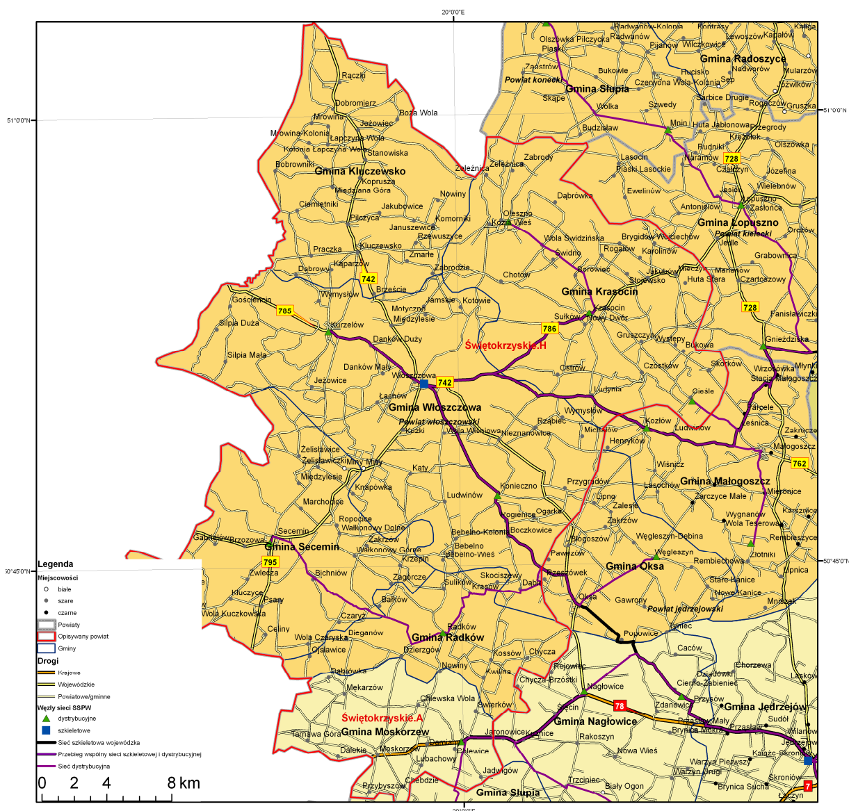
Rysunek 21 Wizualizacja przebiegu sieci szkieletowej i dystrybucyjnej w powiecie włoszczowskim
