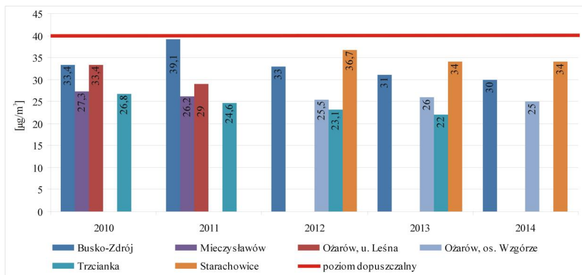
Rysunek 10. Wyniki pomiarów stężeń średniorocznego pyłu PM 10 na stanowiskach pomiarowych w strefie świętokrzyskiej w latach 2010-2014 31
