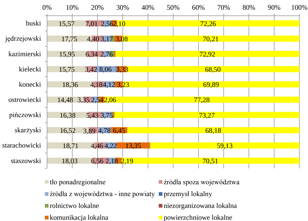
Rysunek 27. Średni udział procentowy grup źródeł emisji w stężeniach średniorocznych pyłu PM 2,5 na obszarze przekroczeń stężeń pyłu PM 2,5 w strefie świętokrzyskiej. 65
