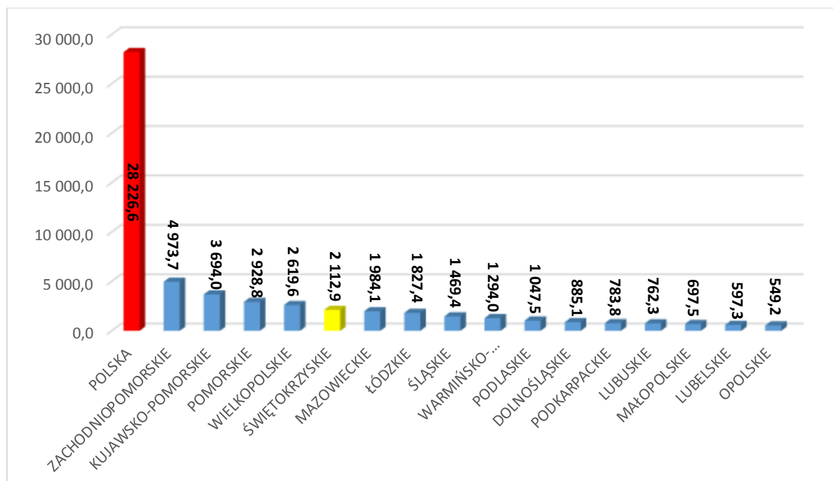
Wykres 58. Produkcja energii elektrycznej z odnawialnych nośników energii ogółem wg województw w 2020 r. w GWh
