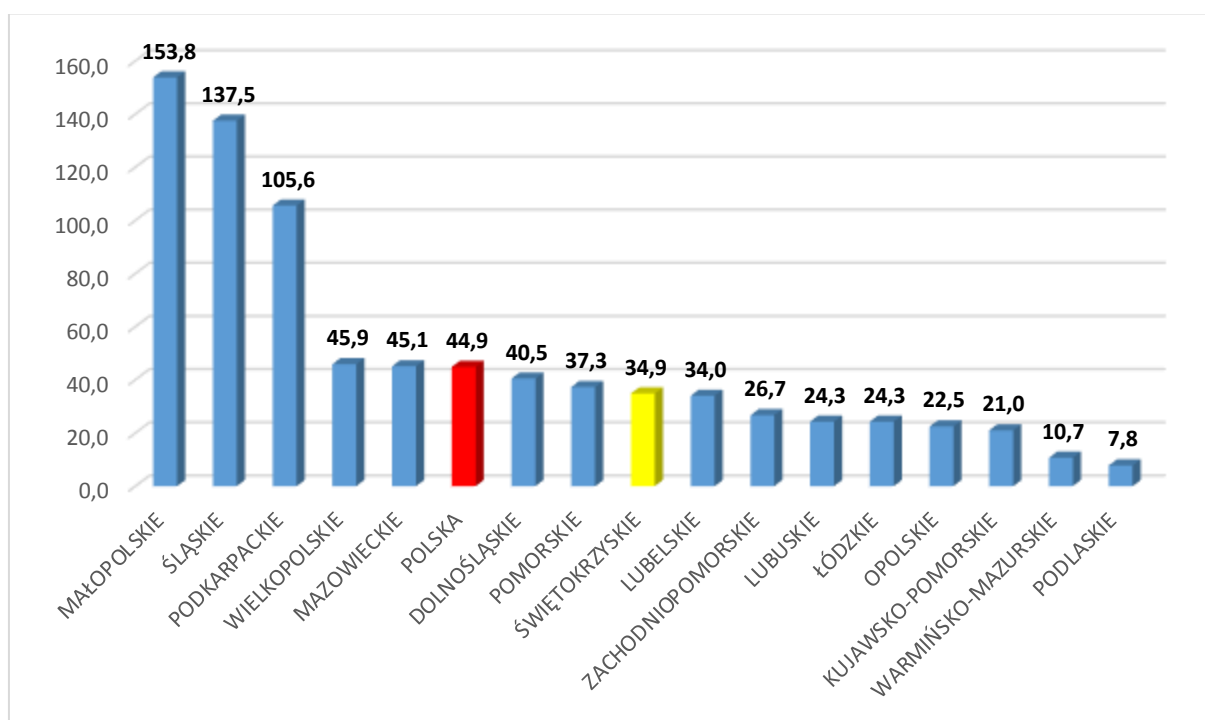
Wykres 64. Sieć rozdzielcza gazowa na 100 km 2 w 2020 roku
